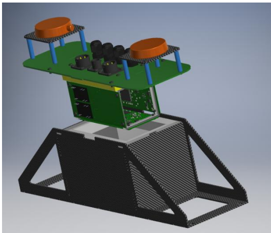
Abbildung 1: Elektronikeinheit
