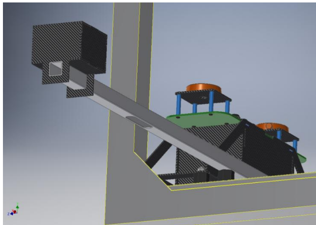
Abbildung 2: Sensorausleger
